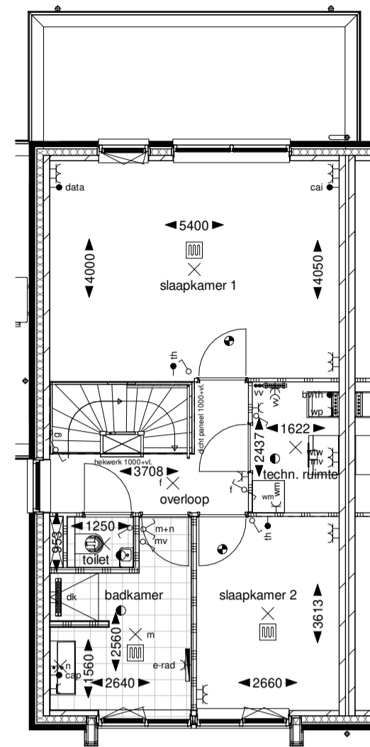
Eerste verdieping
