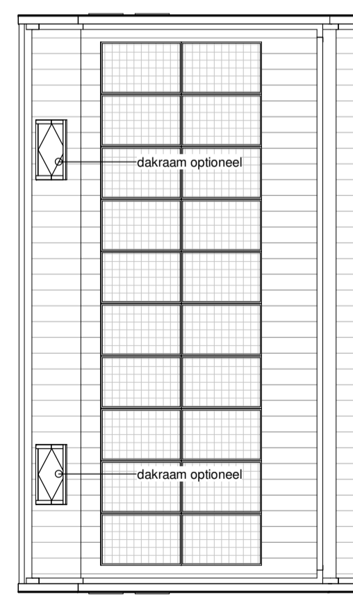
Dakaanzicht
