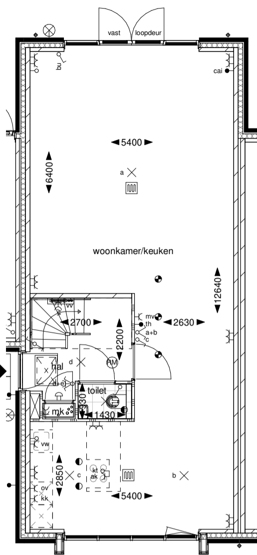
Begane grond
