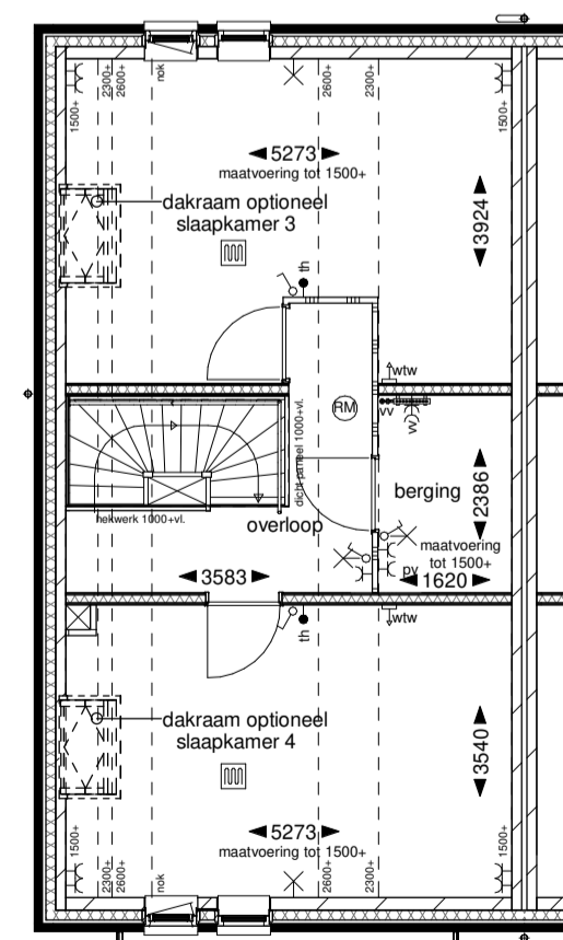
Tweede verdieping
