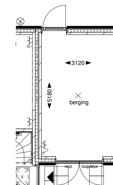
Begane grond
