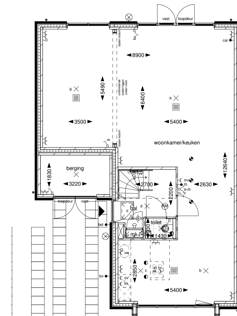
Begane grond
