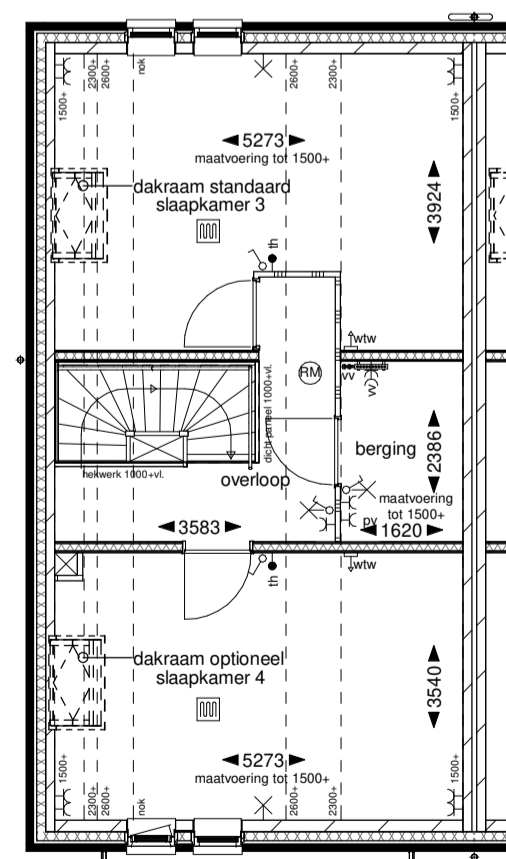
Tweede verdieping
