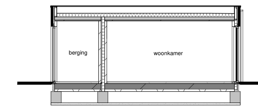
Doorsnede
